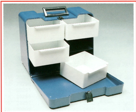
Cassetta per attrezzi - Box for tools Box für Werkzeuge - Caisse pour outils Art. 20810 mm. 475x180x360 h. Art. 20812 mm. 340x180x280 h.
