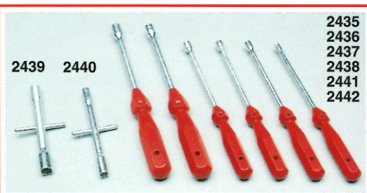
Chiavi a tubo - Nut wrench Mutter-Schlüssel - Clé pour écrou Art. 2439 8 - 10 mm Art. 2440 6 - 7 mm Art. 2435 5 mm Art. 2436 6 mm Art. 2437 7 mm Art. 2438 8 mm Art. 2441 5,5 mm Art. 2442 4 mm
