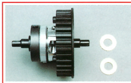
Art. 786007000 Differenziale a sfera - Ball main differential Haupt - Kugeldifferential - Différentiel à billes
