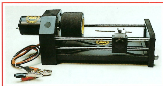
Art. 20950 Microtornio elettrico da casa e da campo per le gomme degli automodelli. L'elettrotensile permette la rapida sagomatura e rettifica di ogni gomma in spugna. 12 volt.
