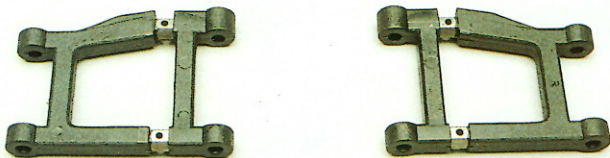
Art. 22596 Kit bracci regolabili - Adjustable arm set
