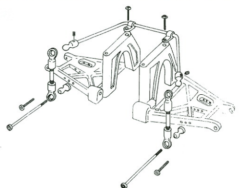
Art. 24302 Set barra stabilizzatrice posteriore Set of rear stabilizer Stabilisator, hinten, Satz
